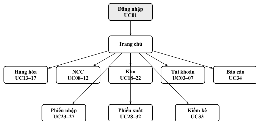
Hình 1: Sơ đồ điều hướng màn hình (menu theo vai trò: QTV chủ yếu Tài khoản)
